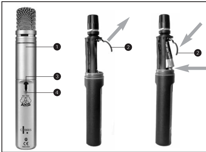
Fig. 1: Introducir la pila
