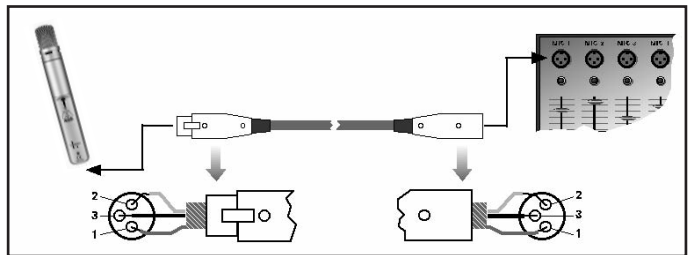
Fig. 4: Collegamento ad uscita simmetrica con alimentazione phantom
